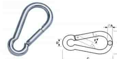
DR-Z0021 SNAP HOOK DIN 5299 FORM C
